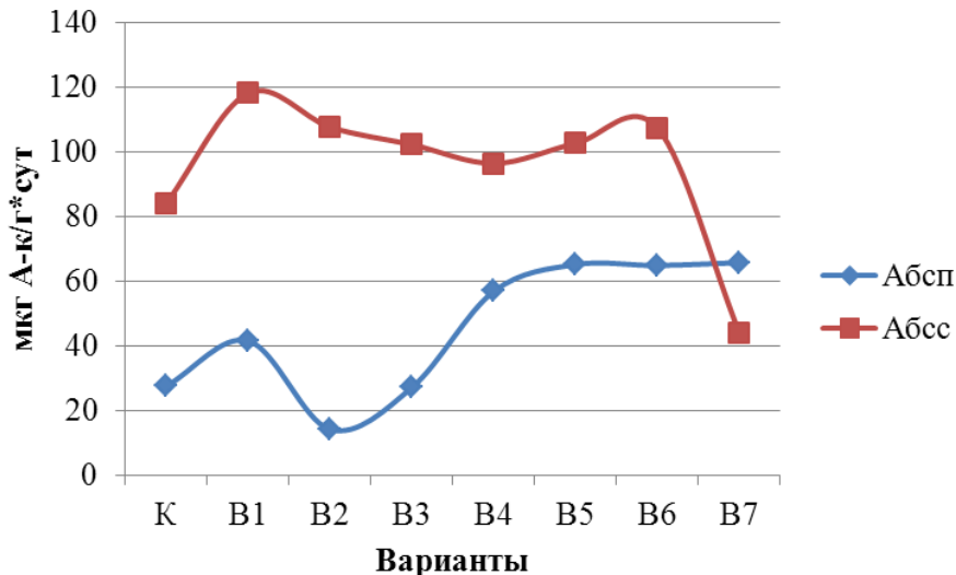
Рис. 3. Протеазная активность A_6 почвы при разном остаточном содержании нефтепродуктов
