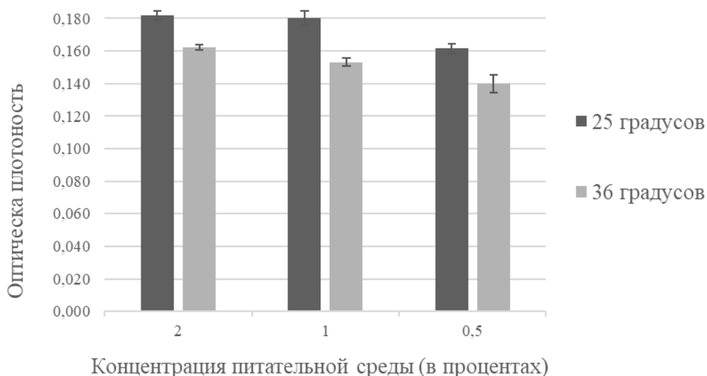
Рис. 1. Оптическая плотность контрольных образцов культуры водоросли хлорелла после 45 часов культивирования при 25 °С и 22 часов при 36 °С в 2, 1 и 0,5 % среде Тамия
