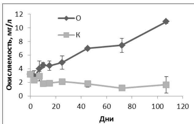
Рис. 1. Изменение содержания легкоокисляемых органических веществ в воде по перманганатной окисляемости
