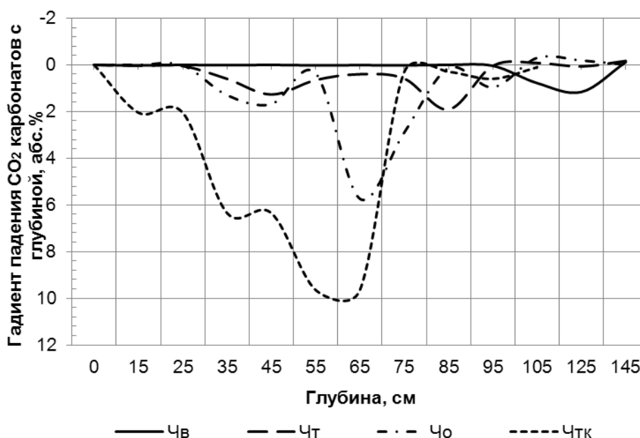
Рис. 1. Распределение градиента падения \text{CO}_2 карбонатов в почвенном профиле черноземов
