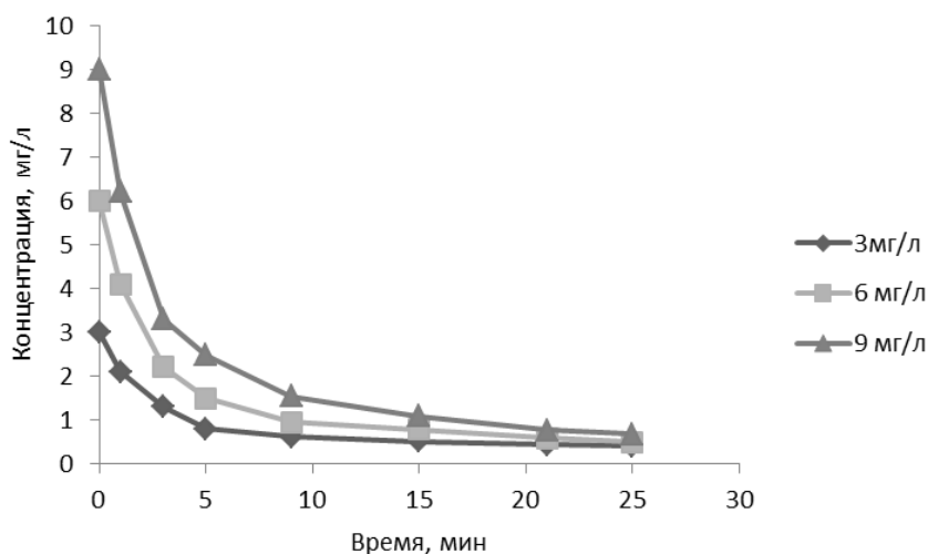
Рис. 2. Зависимость концентрации красителя Black PN
