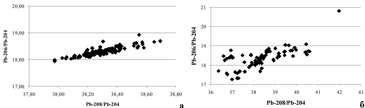
Рис. 2. Трехизотопные диаграммы для различных городов: а – Тюмень, Магнитогорск и Уфа; б – Челябинск и Нижний Тагил
