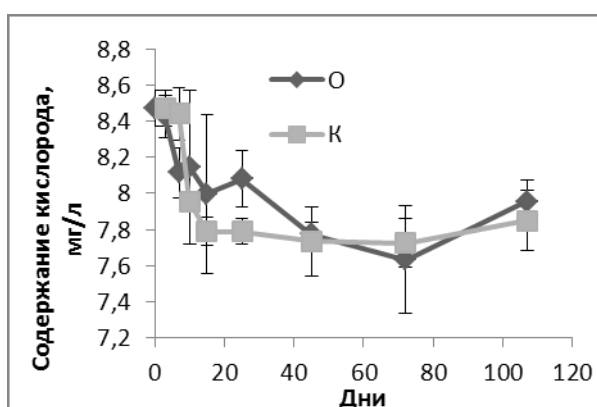
Рис. 2. Изменение содержания растворенного кислорода в воде
