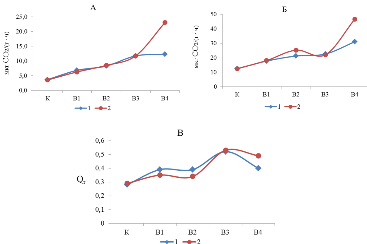
Рис. 1. Параметры дыхательной активности нефтезагрязненной серой лесной почвы: А – V_{\text{базал}} ; V_{\text{сид}} ; В – Q_r : 1 – без удобрения; 2 – с аммофоской
