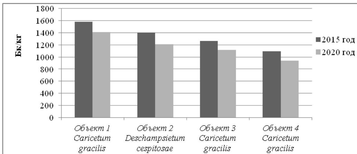
Рис. 1. Удельная активность ^{137}\text{Cs} в почве луговых экосистем в пойме р. Беседь Ветковского района в 2015 г. и 2020 г.
