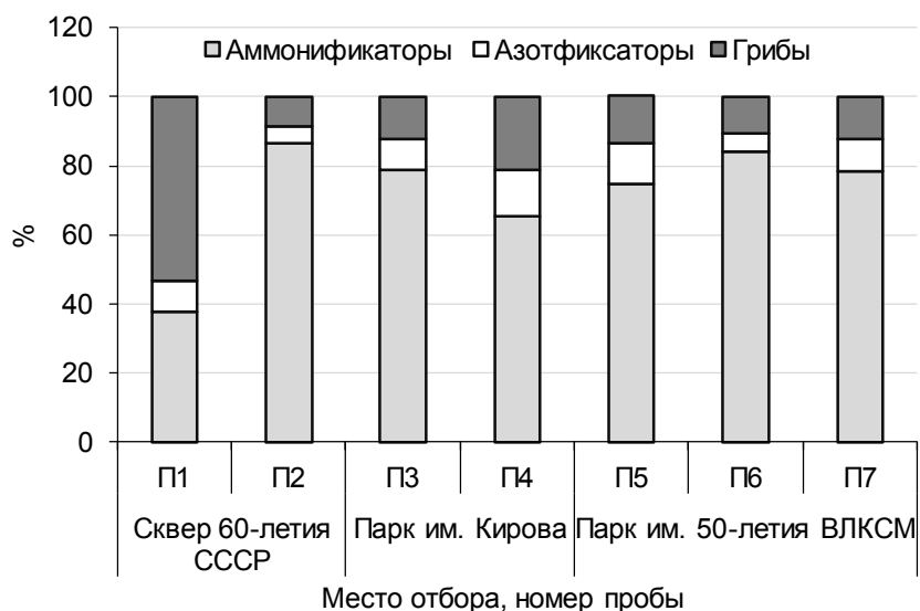
Рис. 2. Структура микробных популяций в урбаноземах парков г. Кирова (%)
