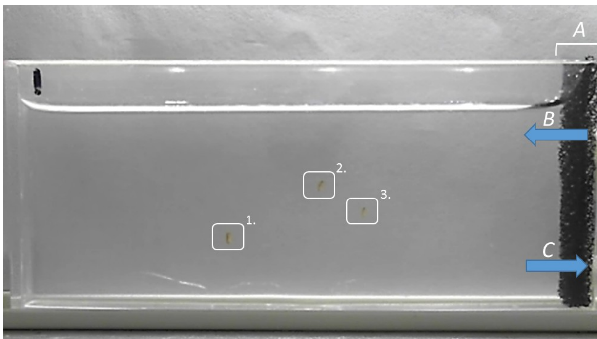
Рис. 1. Проточная тестовая камера во время выполнения эксперимента. 1, 2, 3 – дафнии; А – защитный водопроницаемый слой, В – поступление воды, С – отток воды
