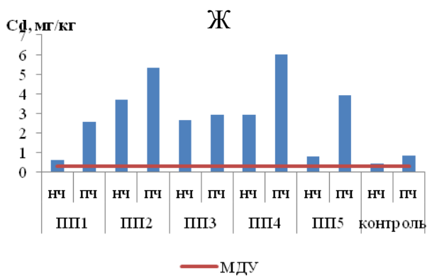
Рис. Диапазон содержания тяжелых металлов в укусах биомассы растительности (нч – надземная часть, пч – подземная часть)
