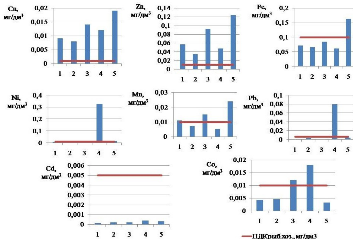
Рис. 2. Содержание тяжелых металлов в воде реки Худолаз
