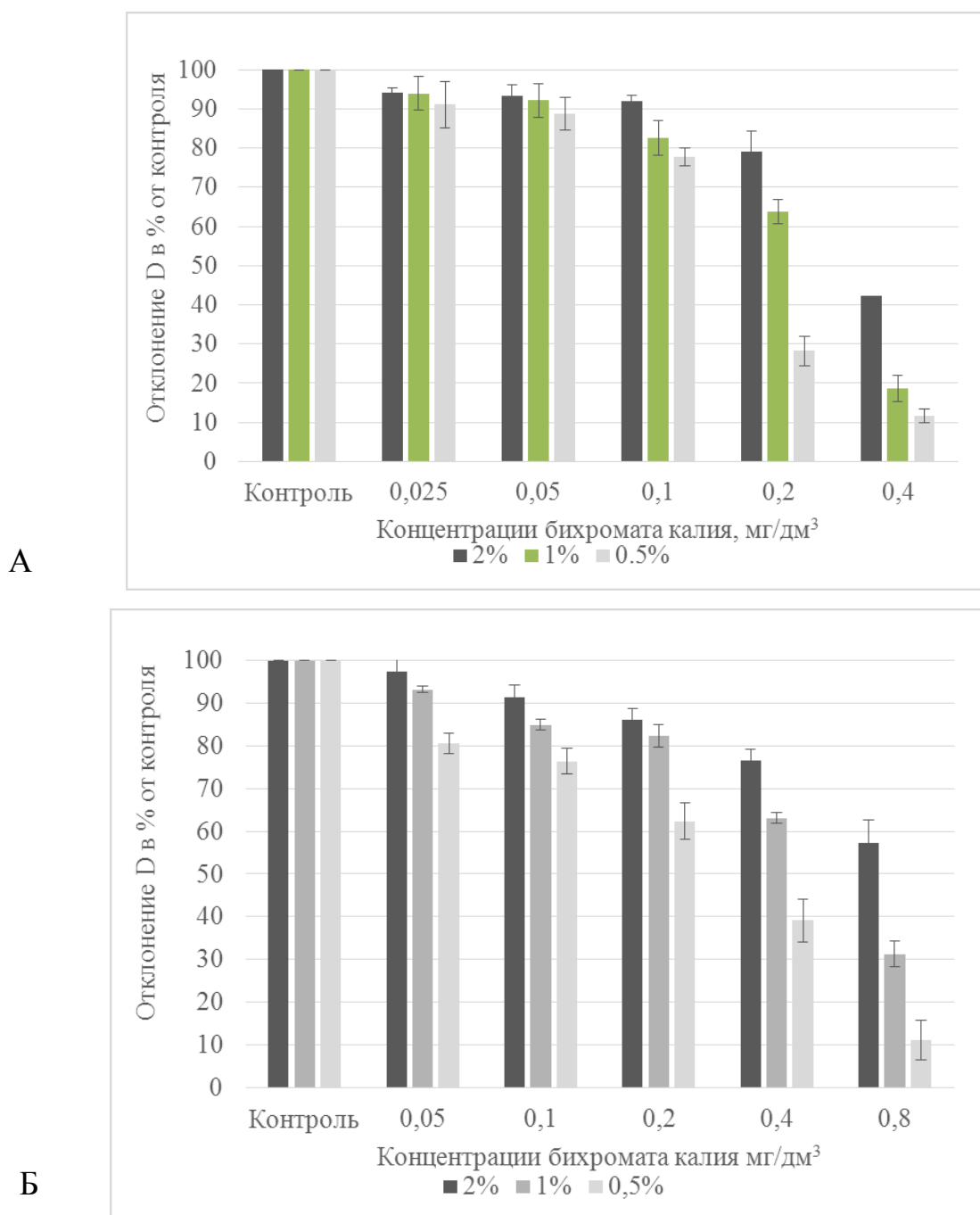
Рис. 2. Отклонение величины оптической плотности (D) суспензии водоросли хлорелла в процентах от контрольного варианта после культивирования при температуре 25 °С (А) и 36 °С в среде Тамия (2, 1 и 0,5%) в присутствии различных концентраций бихромата калия
