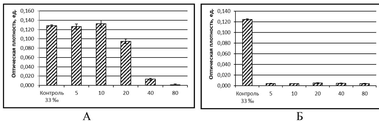
Рис. 2. Оптическая плотность культуры водоросли Dunaliella tertiolecta после 48 часов культивирования на среде Гольдберга в искусственной морской воде 33 ‰ (А) и дистиллированной воде (Б) в присутствии различных концентраций KCl (в г/дм 3 )
