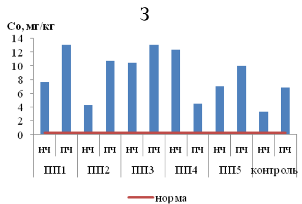
Рис. Диапазон содержания тяжелых металлов в укусах биомассы растительности (нч – надземная часть, пч – подземная часть)
