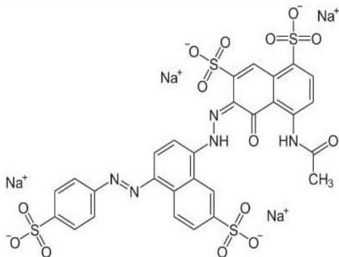
Рис. 1. Структурная формула красителя Black PN
