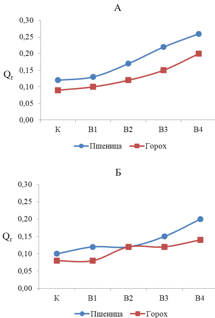
Рис. 2. Коэффициент микробного дыхания ( Q_r ) рекультивированной Ад почвы под посевами различных культур. А – первичный посев, Б – вторичный посев
