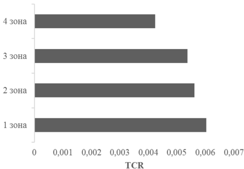
Рис. 1. Суммарный канцерогенный риск (TCR) здоровью взрослых в отдельных зонах г. Казани
