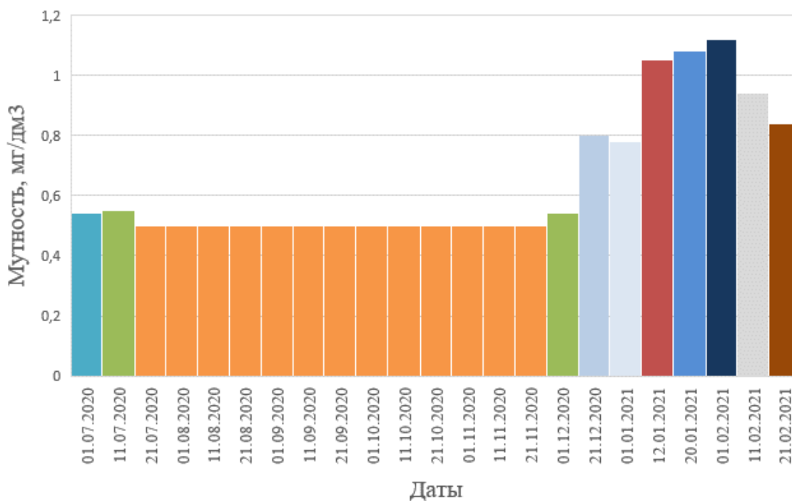
Рис. 2. График изменения мутности в Пионерском водоеме
