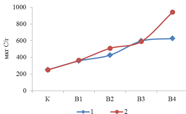
Рис. 2. Содержание микробной биомассы (Смик) в нефтезагрязненной серой лесной почве. 1 – без удобрения; 2 – с аммофоской
