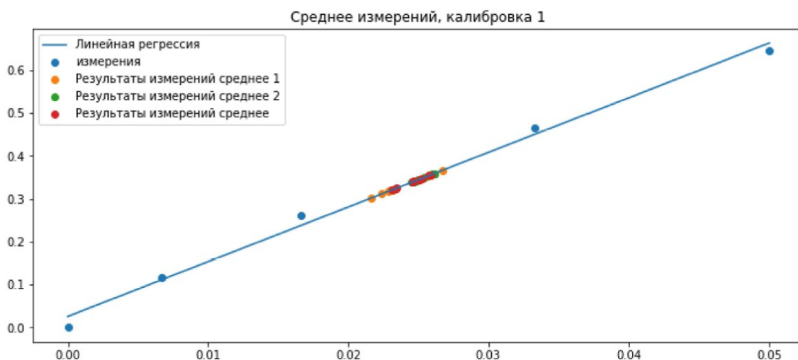
Рис. 1. Градуировочный график для определения активности каталазы
